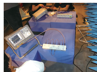
電波暗室での通信実験（専攻科）
