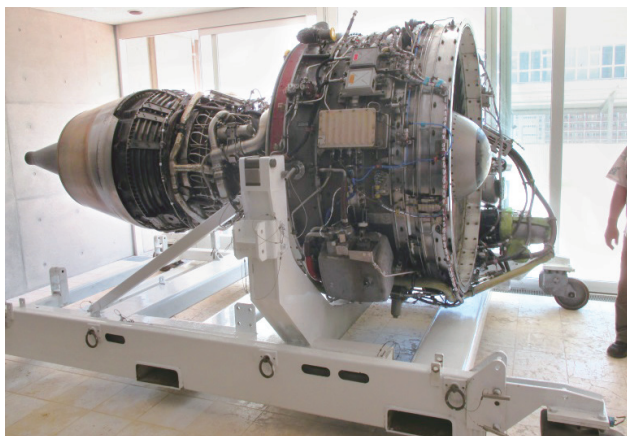
校内に設置されたジェットエンジン（JTA（株）様より寄贈）
