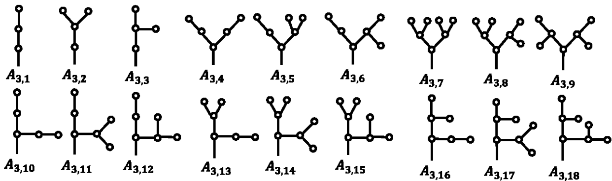
図3 3年目のポチヨウジのグラフによる分枝モデル
