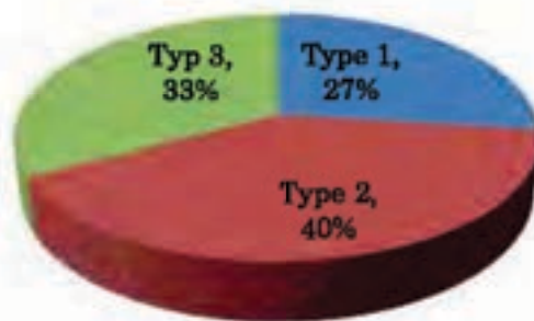
図5 ナガミポチヨウジの分枝発生パターンの割合
