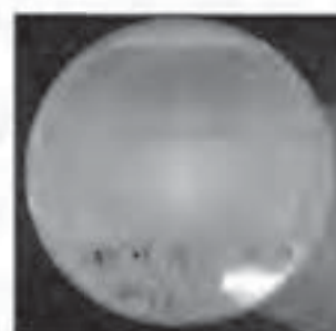
図 2. エピオス培地上の菌糸
