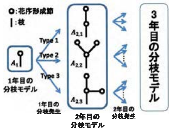
図2 ポチヨウジ属のグラフによる分枝モデル
