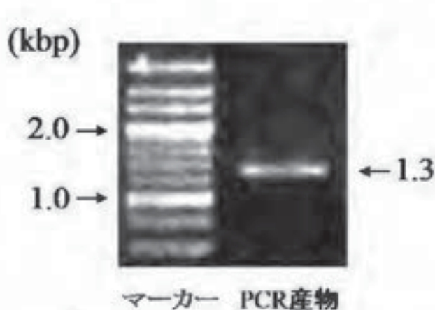
図 4. PCR 産物の電気泳動結果
